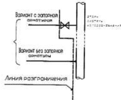
ЭСКИЗ № 5
